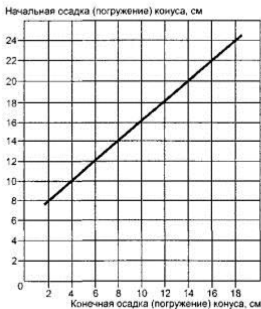
Рисунок 1 - Критерий сохраняемости подвижности
